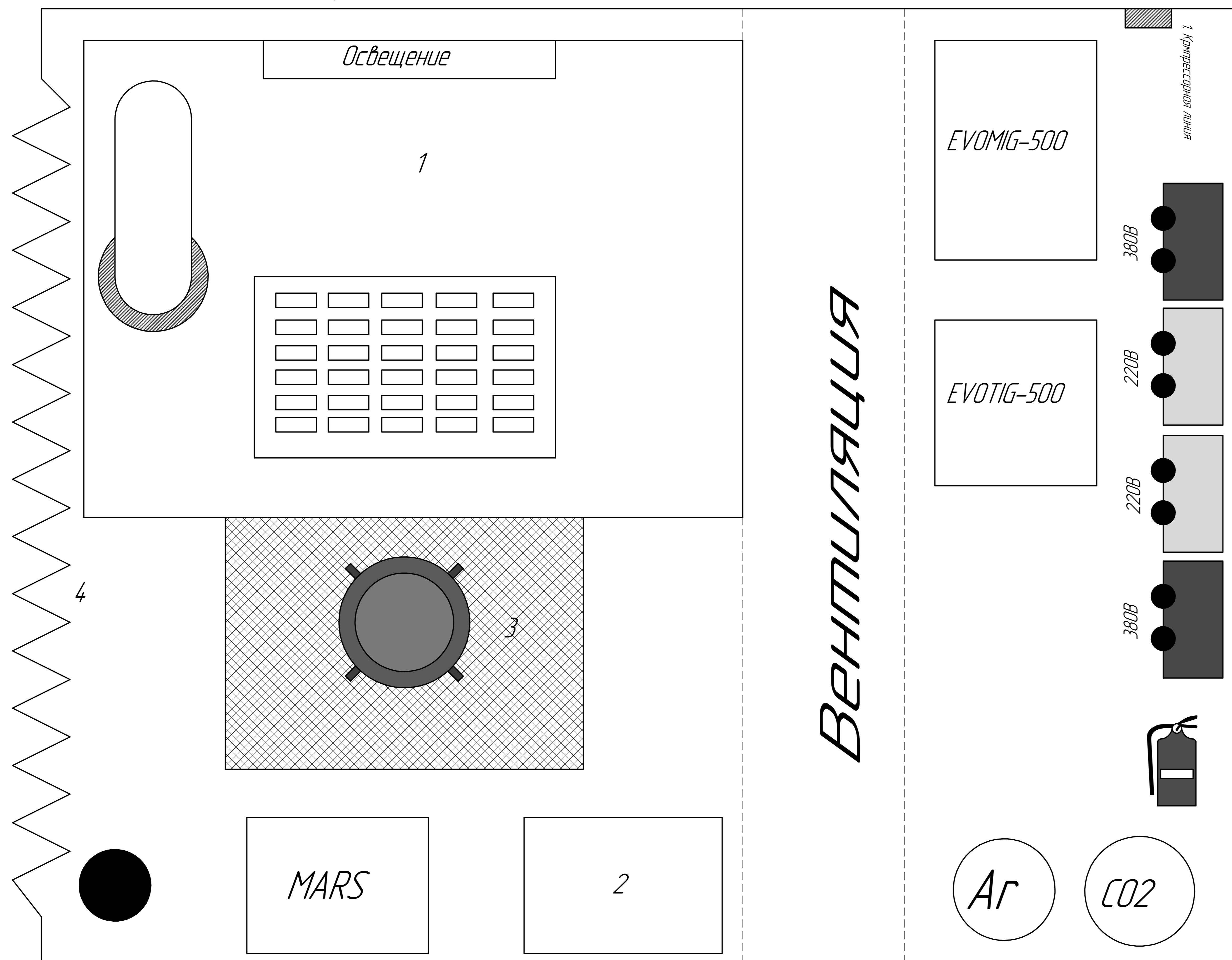
Сварочный пост 2
